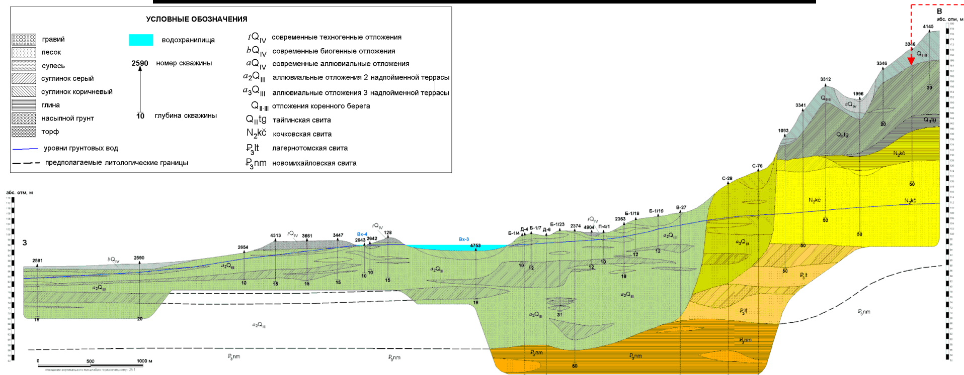
Рисунок 4.6- Инженерно-геологический разрез через модульные сооружения ППЗРО
