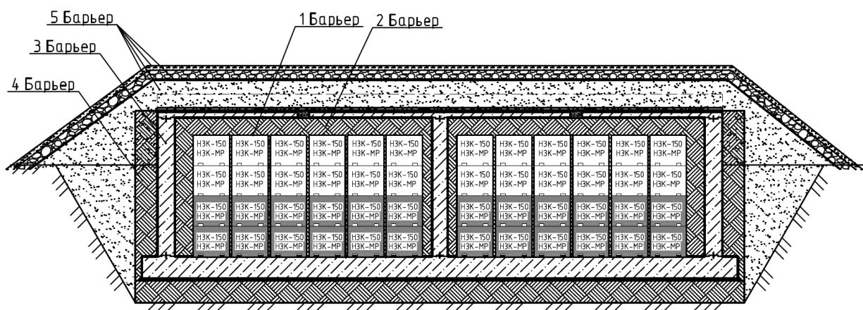
Рисунок 3.4 – Конструкция барьеров защитного покрывающего экрана
