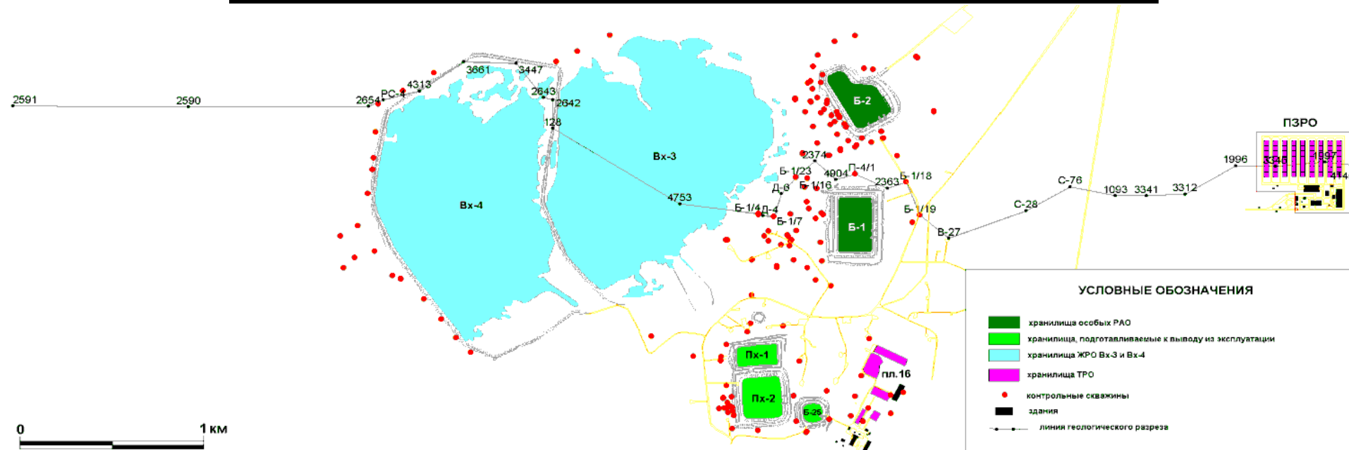
Рисунок 4.7- Геологический разрез района размещения ППЗРО
