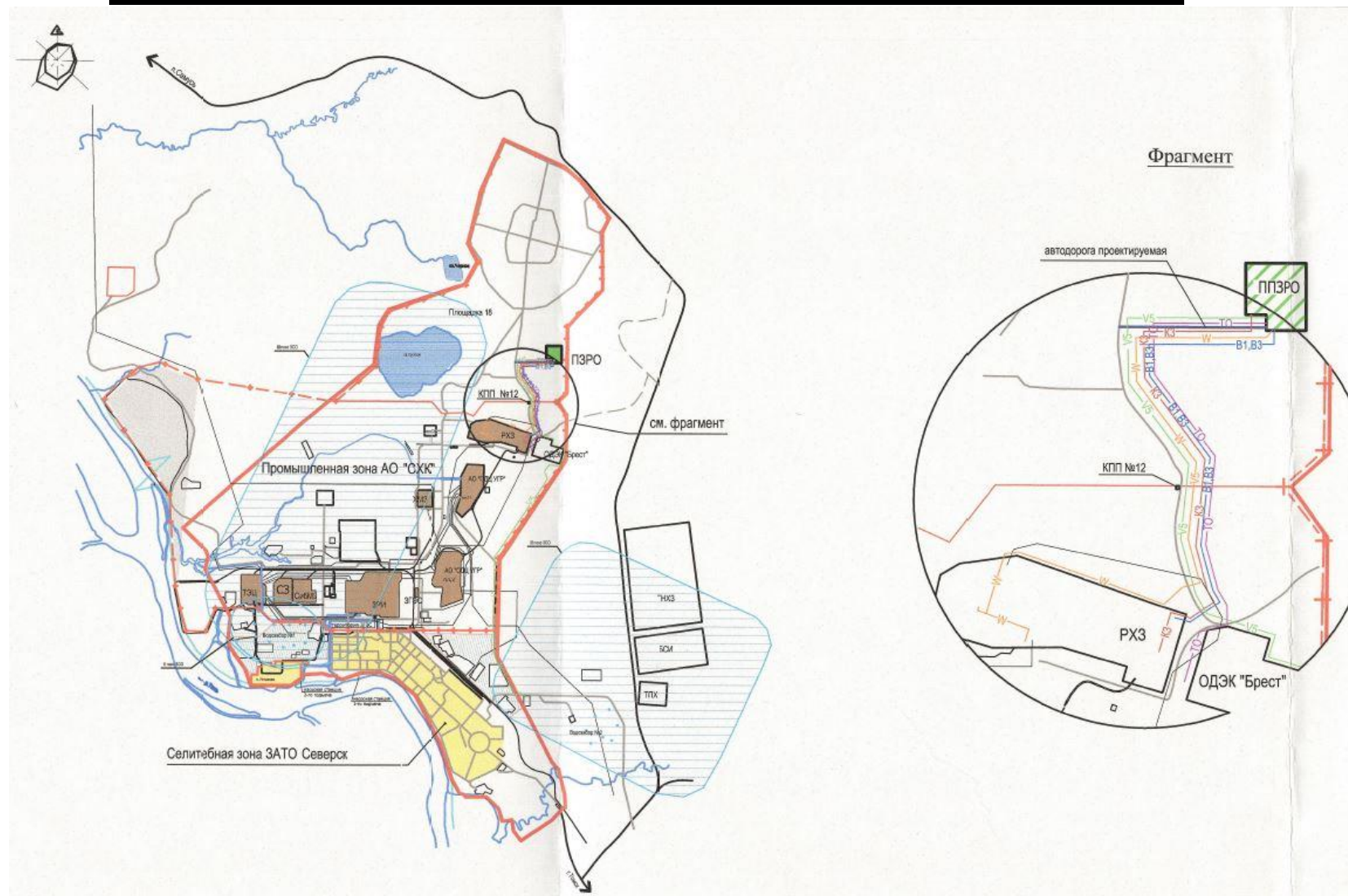
Рисунок 3.2 – Ситуационная схема размещения площадки ППЗРО
